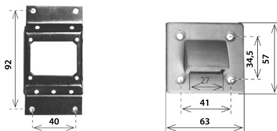
GUIDACINGHIA IN NYLON BIANCO per cassonetto prefabbricato e supporto in ferro
