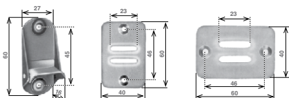
passacinghia e bloccacinghia per avvolgitore Omega
