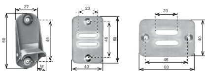
passacinghia e bloccacinghia per avvolgitore Omega
